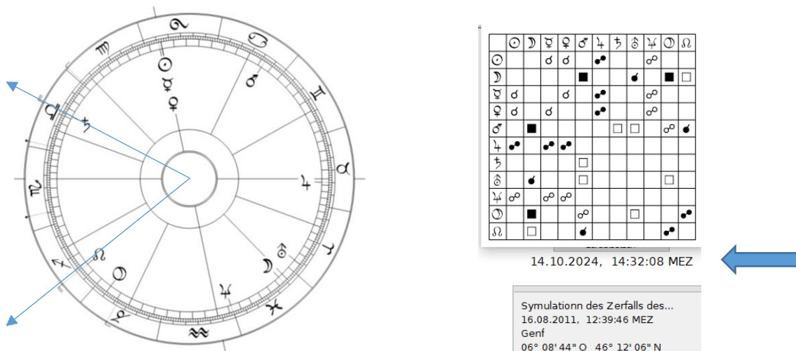
Abb. 3: Veröffentlichung des Modells der Synchronisation des Zerfalls des Higgs-Teilchens. (siehe Abb. 1/S. 8).
