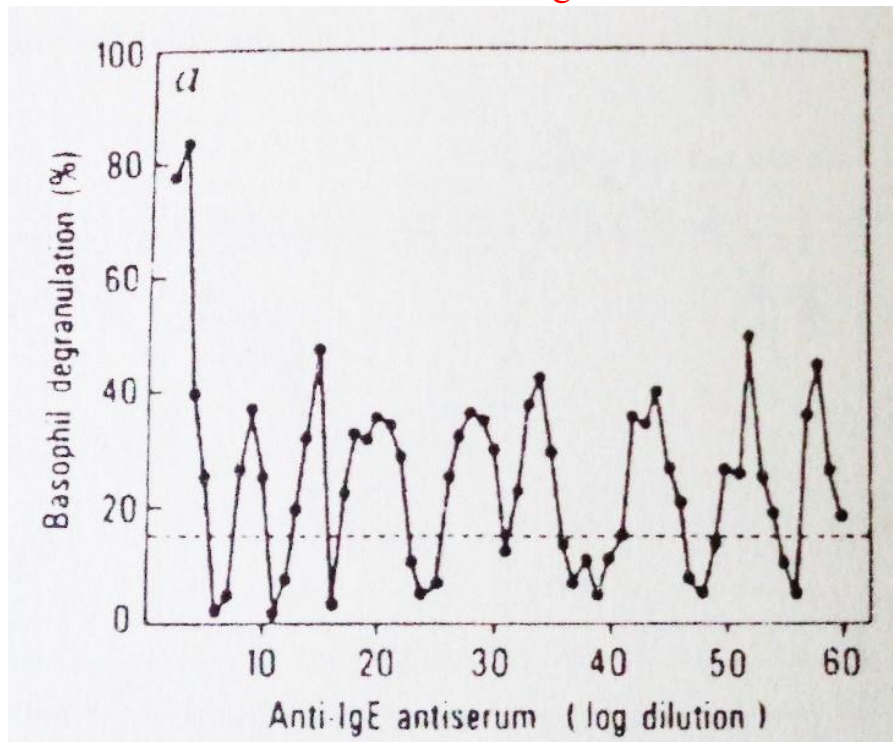
Abb. 1: Degranulation von Abwehrzellen nach Benveniste, 1988. 22
