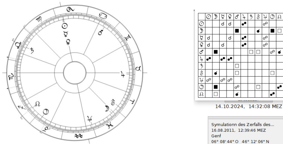
Abb. 1: Veröffentlichung des Modells der Synchronisation des Zerfalls des Higgs-Teilchens. (siehe Abb. 1/S. 8).
