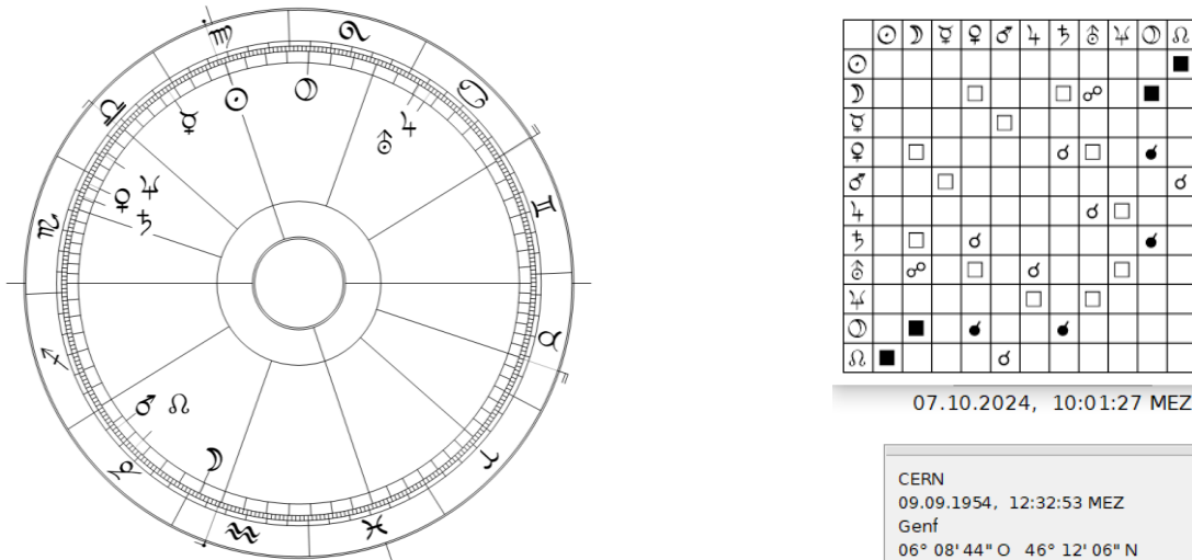
Abb. 1: Gründung der europäischen Organisation für Kernforschung (CERN)
