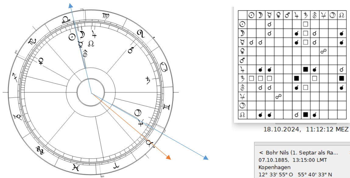
Abb. 1: Nils Bohr. Geboren am 7.10.1885.
